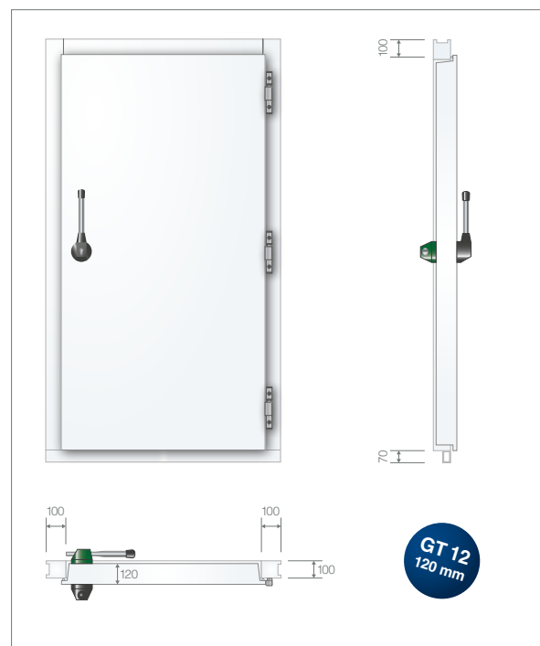
Tiefkühlraumtür GT 12 120 mm Isolierstärke, + 25° C bis - 30° C Standardblockrahmen für den Einbau in Mauerwerk
