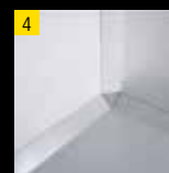
Edelstahlboden (1.4509), vollhygienisch, kreisverpresst, rutschfest, Flächenlast in kg/m²: 2000
